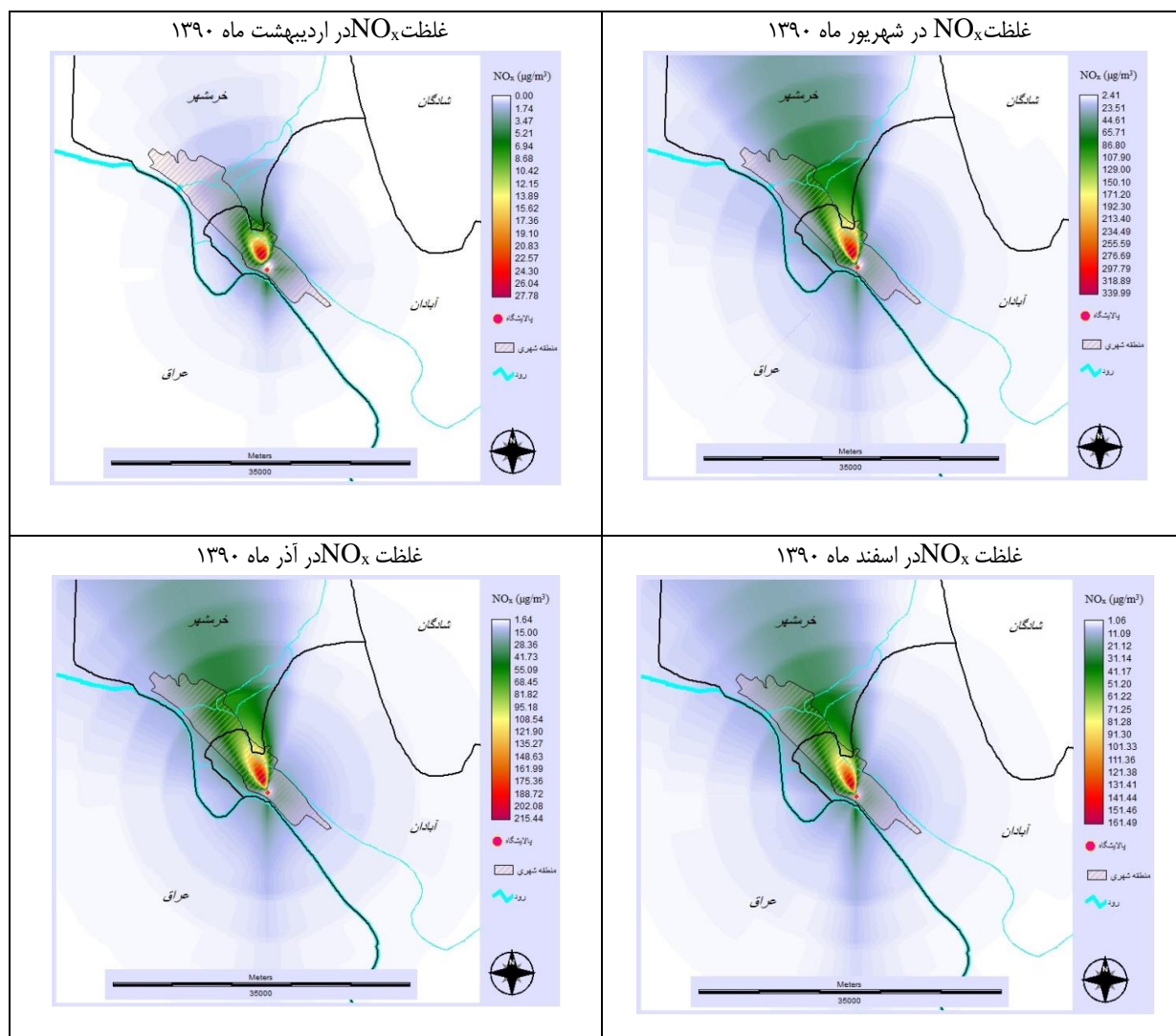
شکل (۳): پراکنش آلودگی NO x پالایشگاه نفت آبادان در ماه‌های مورد مطالعه
