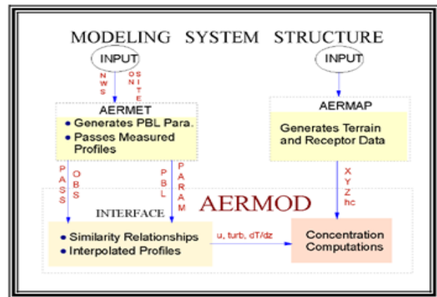
شکل (۱): ساختار کلی مدل AERMOD و رابطه آن با پیش‌پردازنده‌ها (USEPA, 2004)
